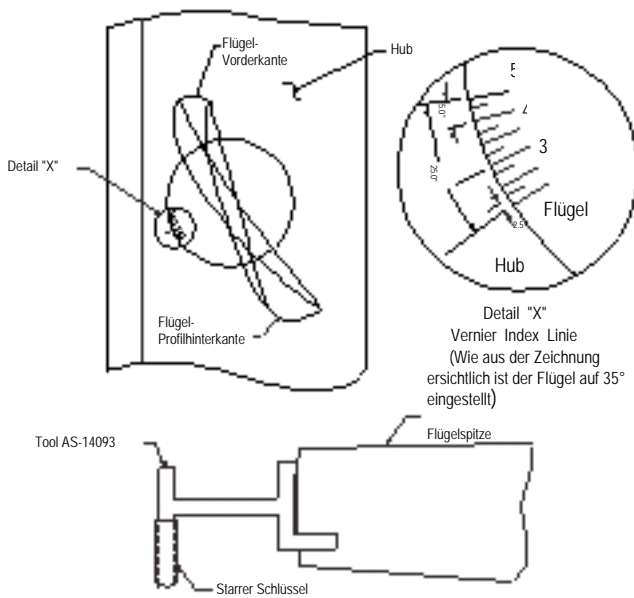
Abbildung 10. TCVX Flügelwinkleinstellung
