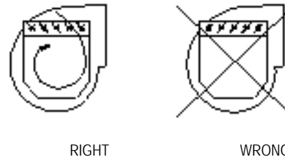
Abbildung 7. Ausrichtung der Dämpferschneiden im Verhältnis zu der Ventilatorrotation
