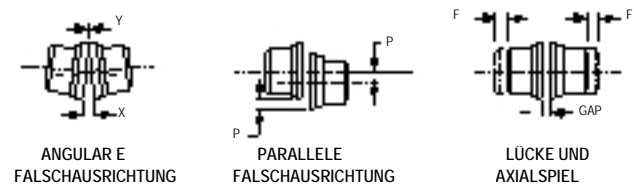
Abbildung 6. Kupplungsausrichtung
