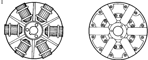
Côté tête et boulon en U
