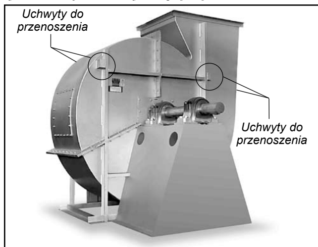
Rysunek 1. Umiejscowienie uchwytów do przenoszenia
