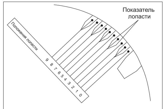
Рис. 13. Маркеры положения лопасти Axiad
